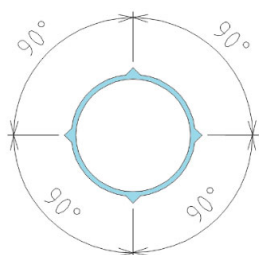
図1 リング断面図 【4ヶ所リブ有り】
